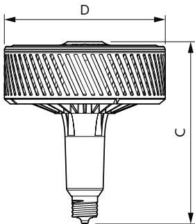
TrueForce LED HPI UN 95W E40 840 NB
