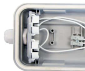
Fassung aufgeklappt (Montagezustand)
