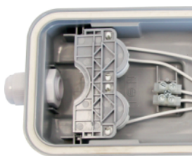
Fassung eingeklappt (Auslieferungszustand)
