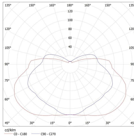
KANLUX S.A. (kat 7025) TURK DL-60 / Krzywa rozsytu światła (biegunowo)
