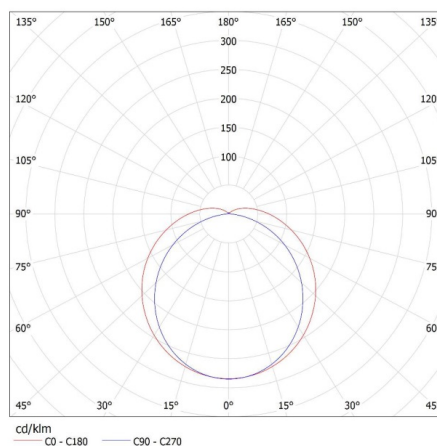
KANLUX S.A. (kat 22603) MAH-LED N 20W-NW / Krzywa rozsyłu światła (biegunowo)
